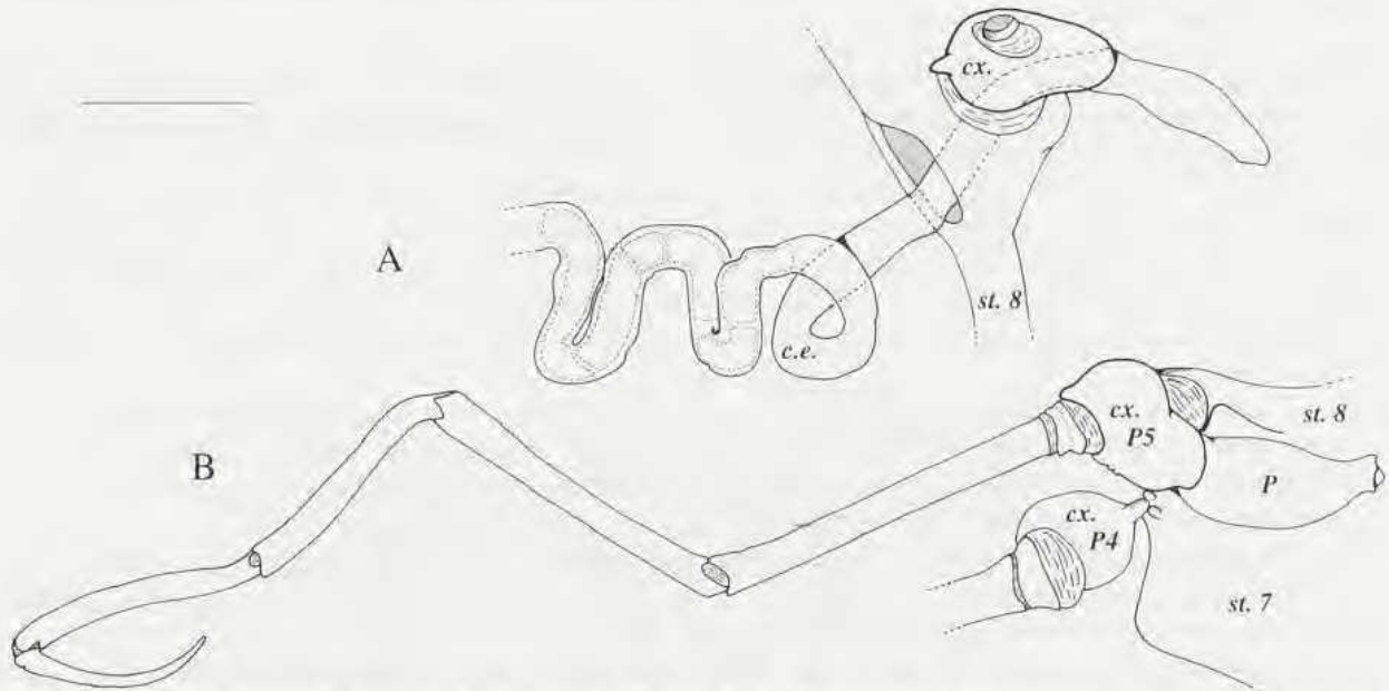
FIG. 1. — Tymolus daviei sp. nov., ♂, BATHUS 2, st. CP 743. A, Trajet du canal éjaculateur qui débouche sur le pénis en passant par la coxa de P5. c.e., canal éjaculateur; cx., coxa de P5 droit; st. 8, sternite 8. — B, vue de la région sternale au niveau des coxae de P4 et P5 droits. cx. P4, cx. P5, coxae de P4 et de P5; P, pénis; st. 8, st. 7, sternites 8 et 7. Échelle = 1 mm.
